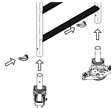
Rys. 33. Montaż zestawu kołowego 150
