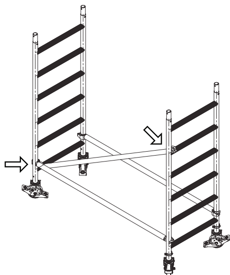
Rys. 54. Montaż stężenia skośnego
